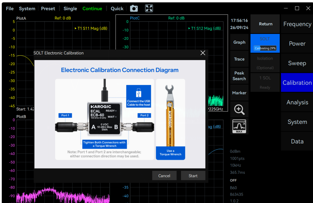
图 7 SOLT 电子校准界面与状态显示
