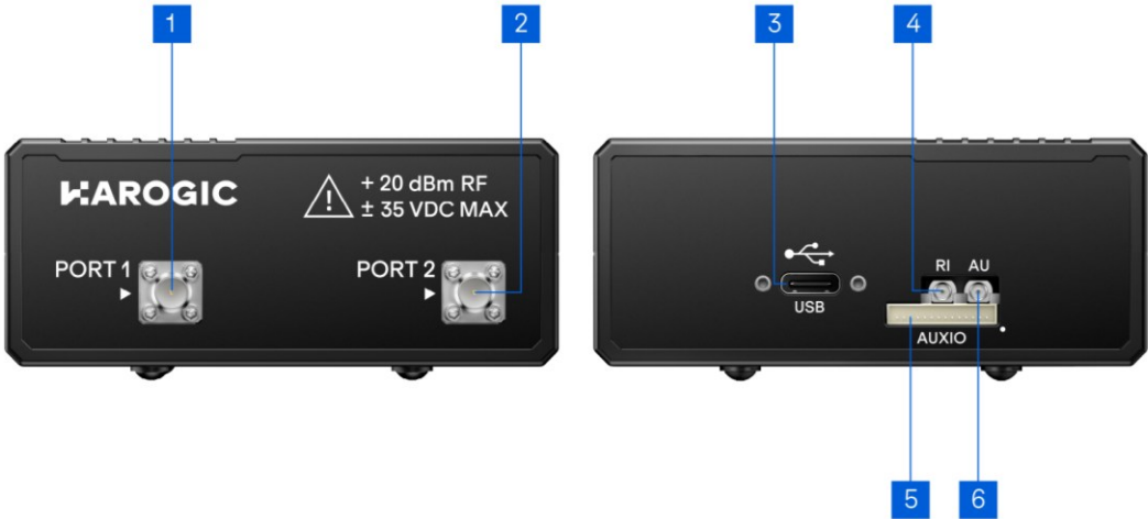
图 1 VNB 系列接口说明
