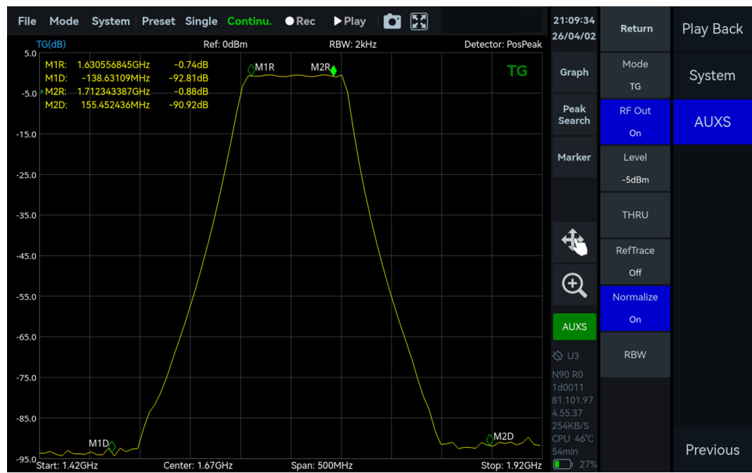
图 50 带通滤波器频率响应曲线
