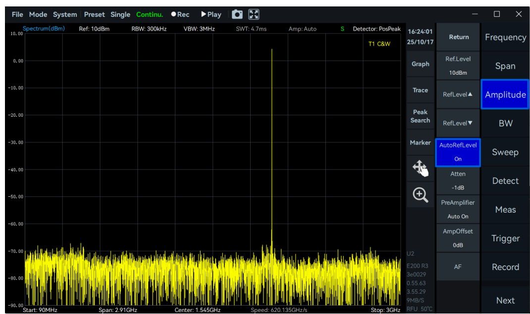
图 29 启用自动参考电平
