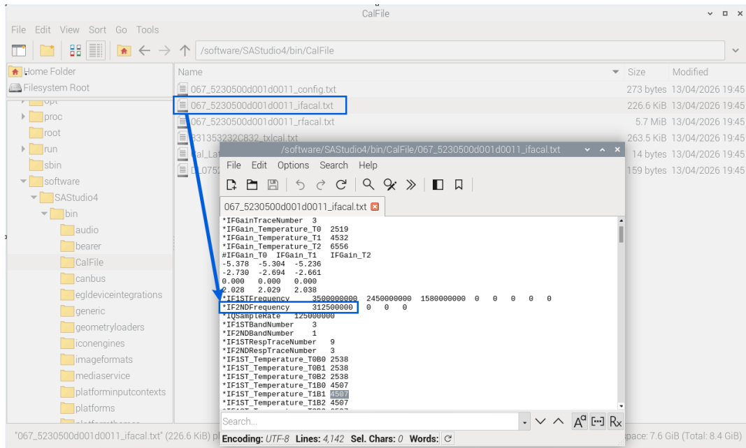
图 53 PX 系列仪器查看中频输出的中心频率
