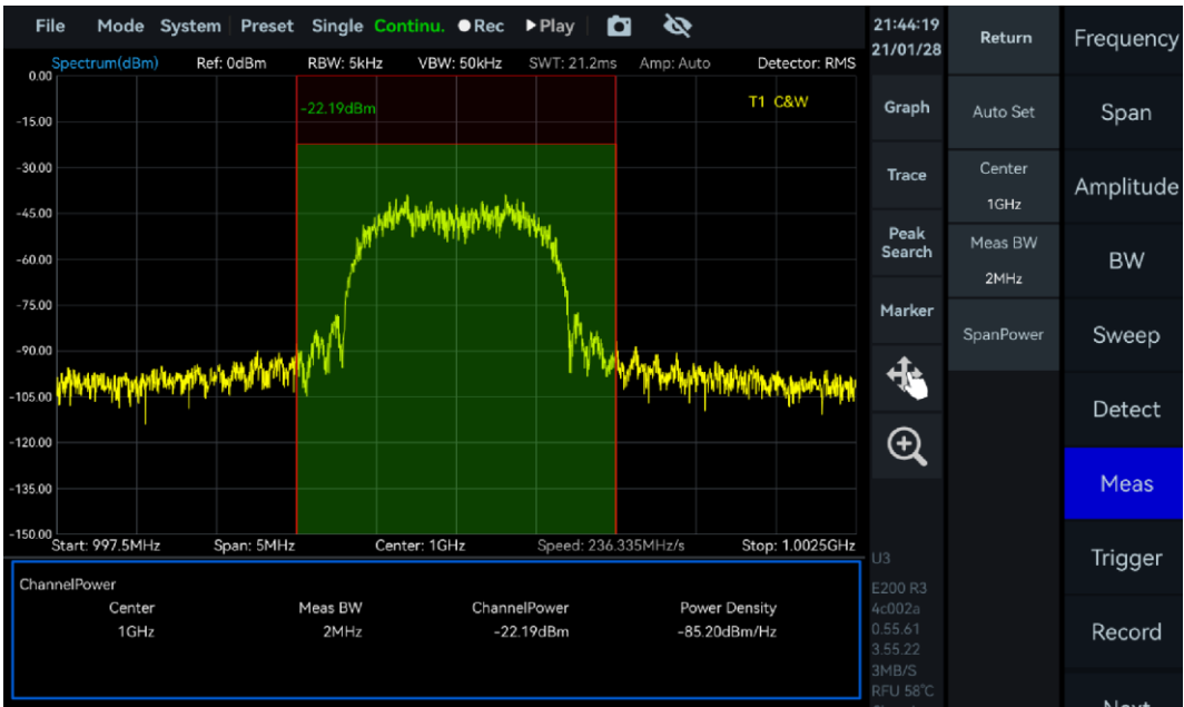
图 24 信道功率测量
