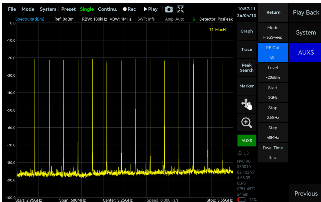
图 49 ASG 输出频率扫描信号
