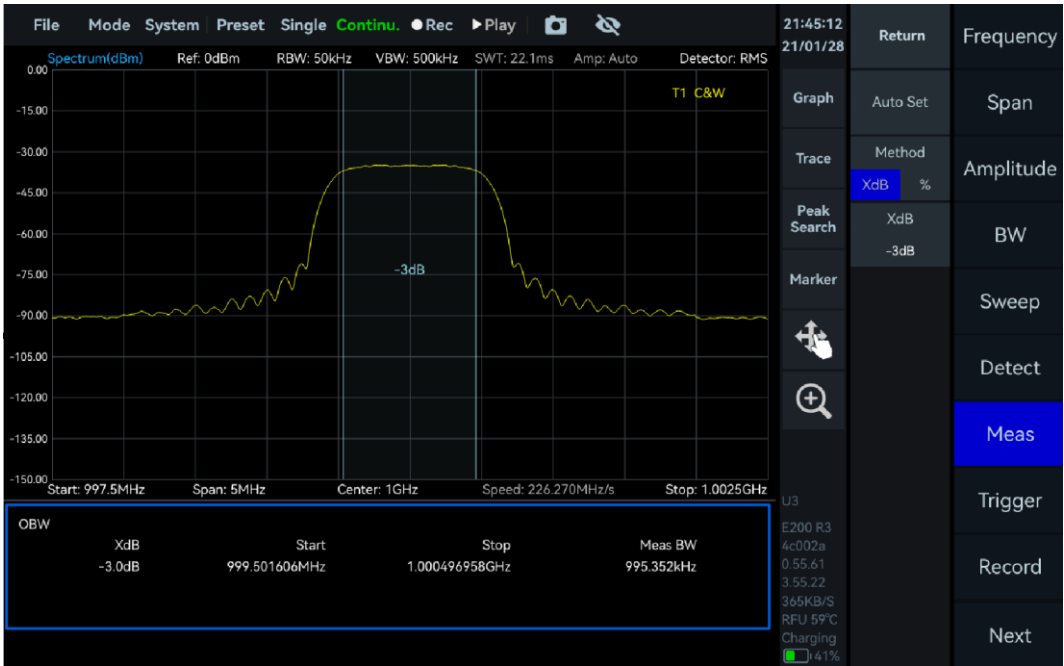
图 25 占用带宽测量
