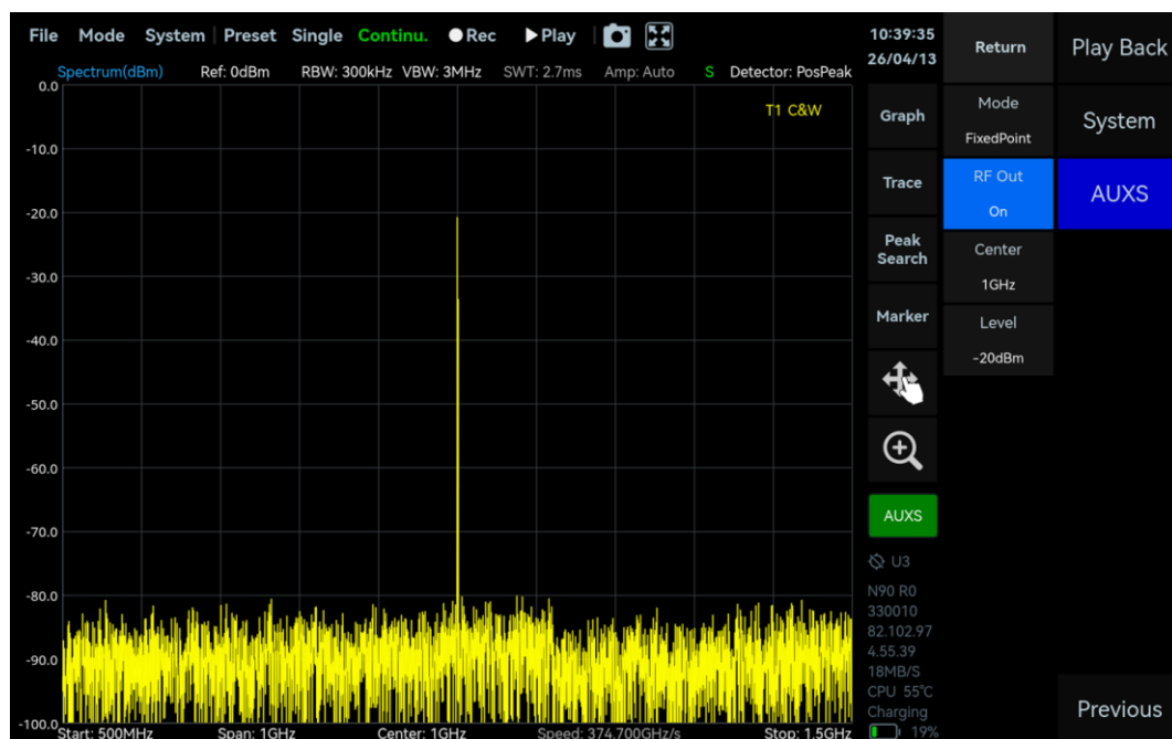
图 48 ASG 输出单音信号
