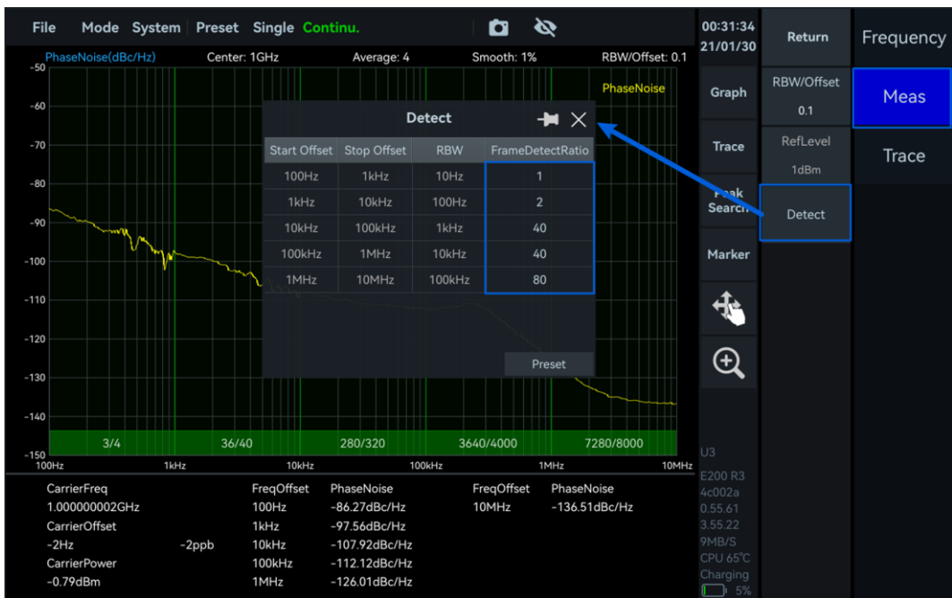
图 46 脉冲信号检测检波设置
