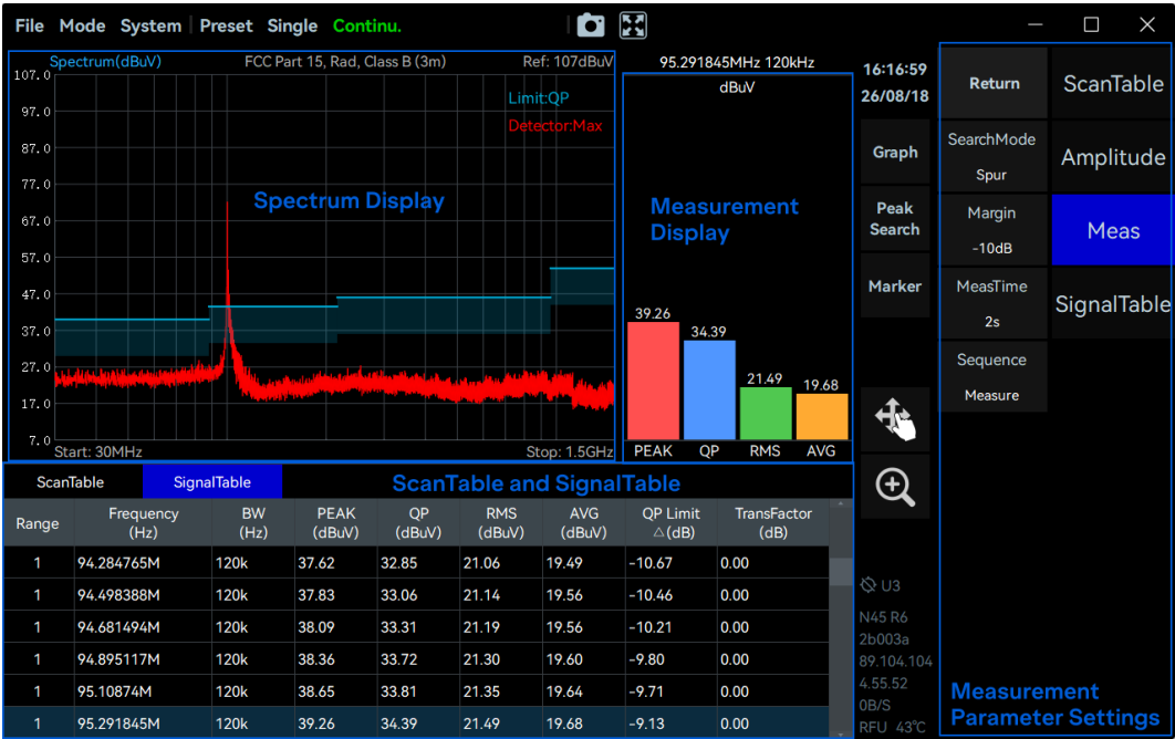
图 51 EMI 预兼容测量界面介绍
