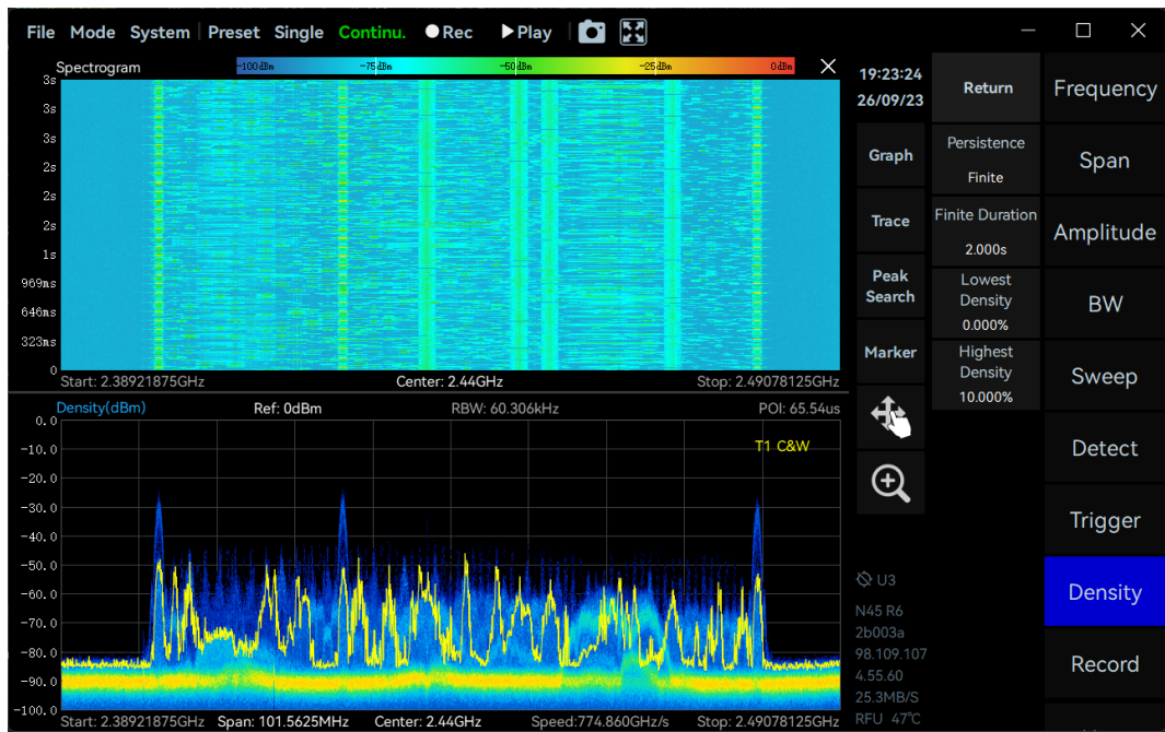
图 43 WIFI 信号的概率密度图
