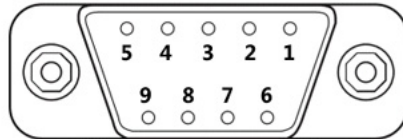
图 9 EIO 拓展板接口示意
