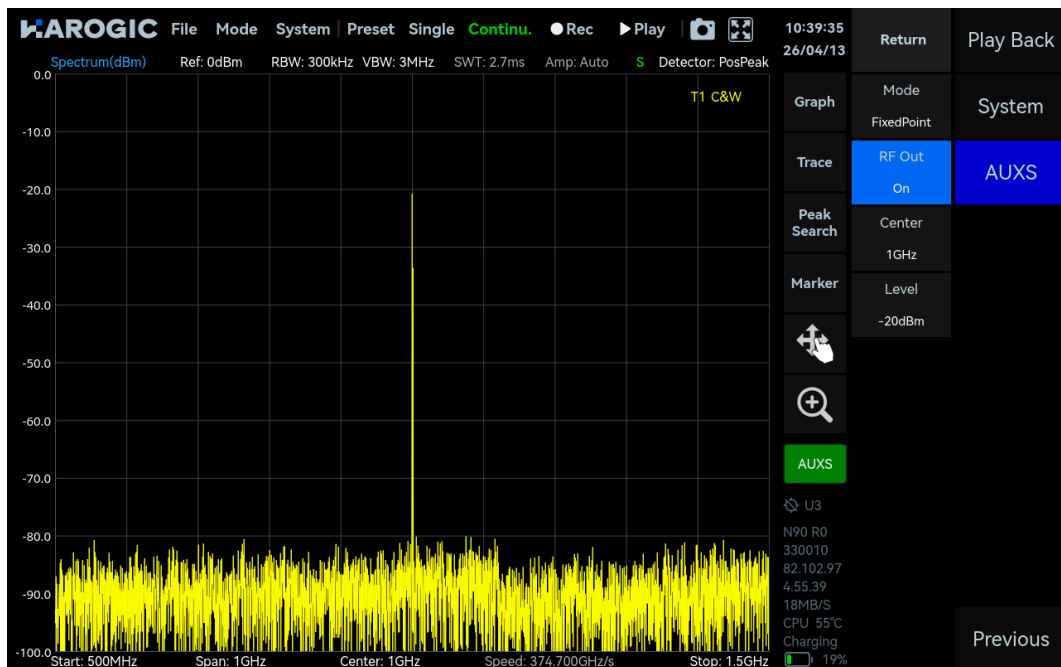
图 46 ASG 输出单音信号
