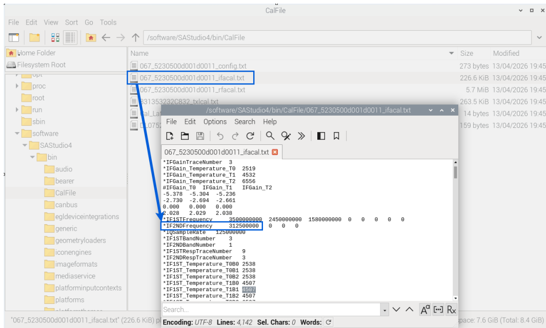
图 49 PX 系列仪器查看中频输出的中心频率
