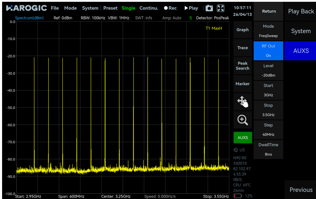
图 47 ASG 输出频率扫描信号
