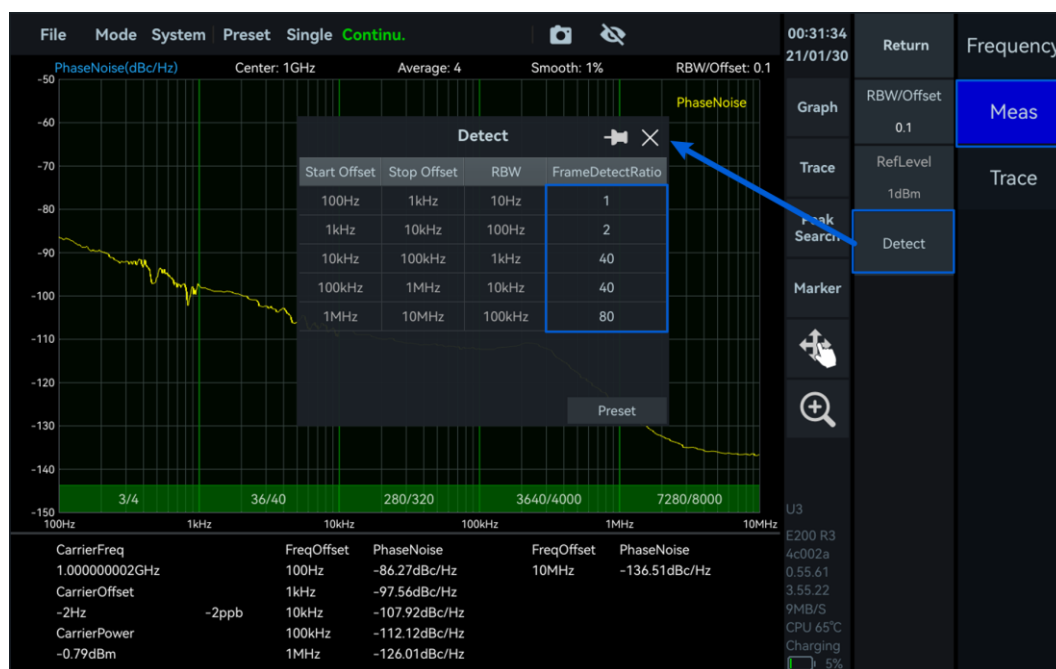
图 41 脉冲信号检测检波设置
