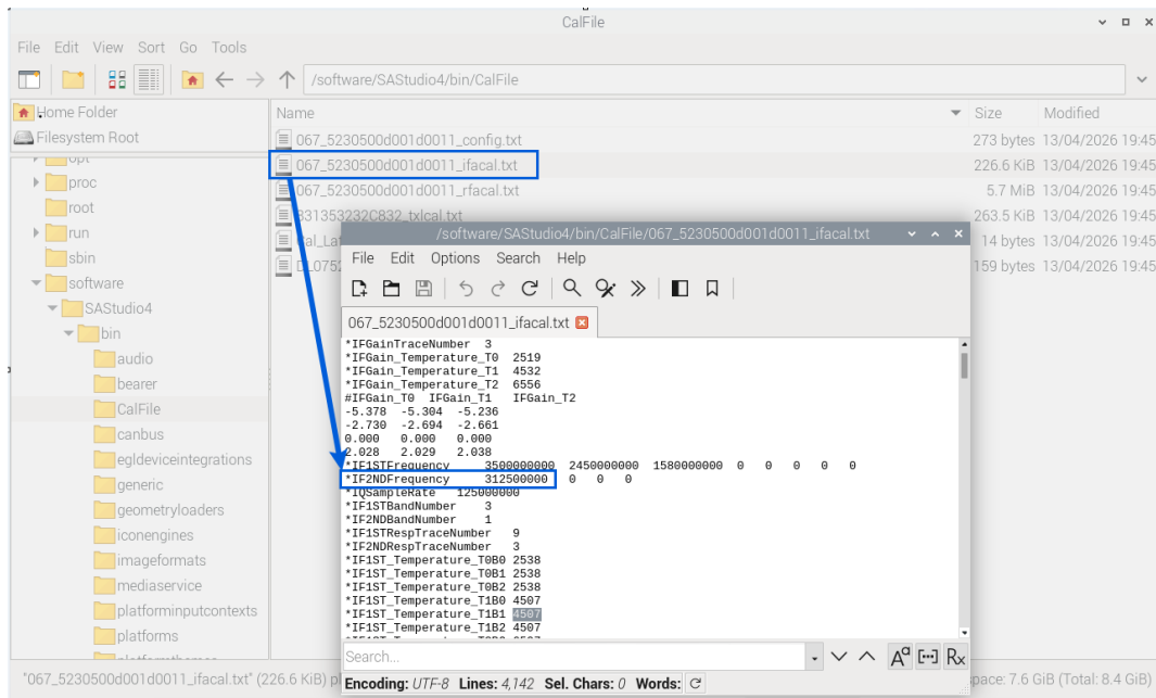
图 47 PX 系列仪器查看中频输出的中心频率
