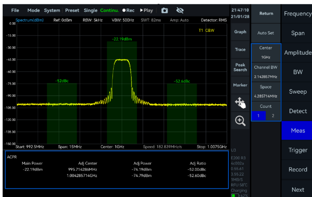
图 21 邻道功率比测量
