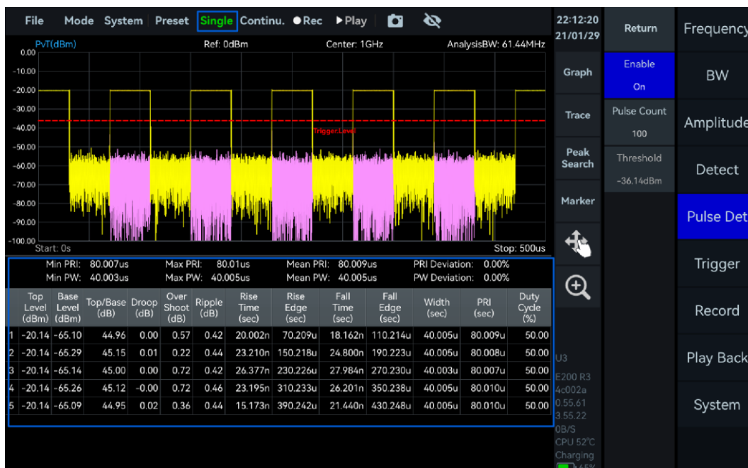
图 36 脉冲检测结果
