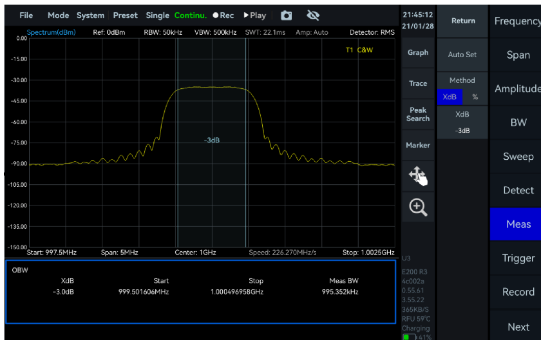
图 20 占用带宽测量
