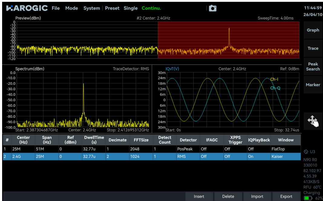
图 43 MSCAN 模式示例
