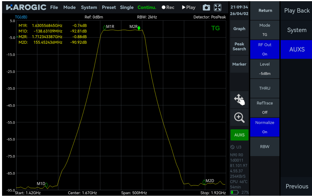
图 46 带通滤波器频率响应曲线
