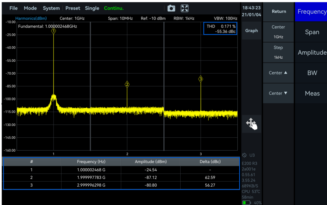
图 40 三次谐波测量
