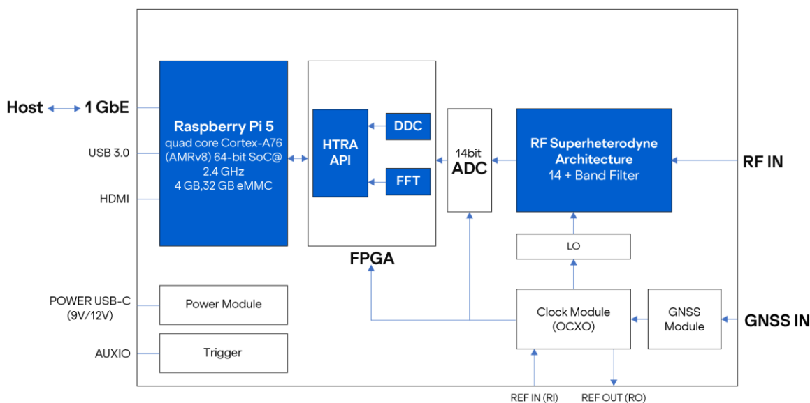
图 3-1 R1000 系列功能级信号流
