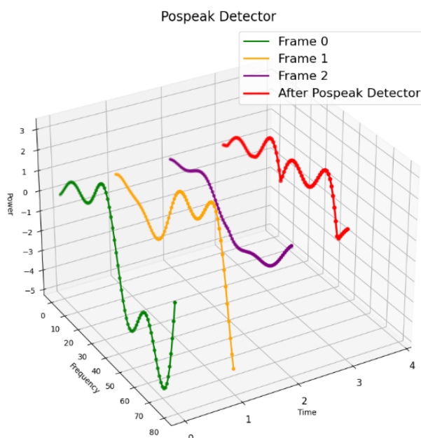
图 9 正峰值检波
