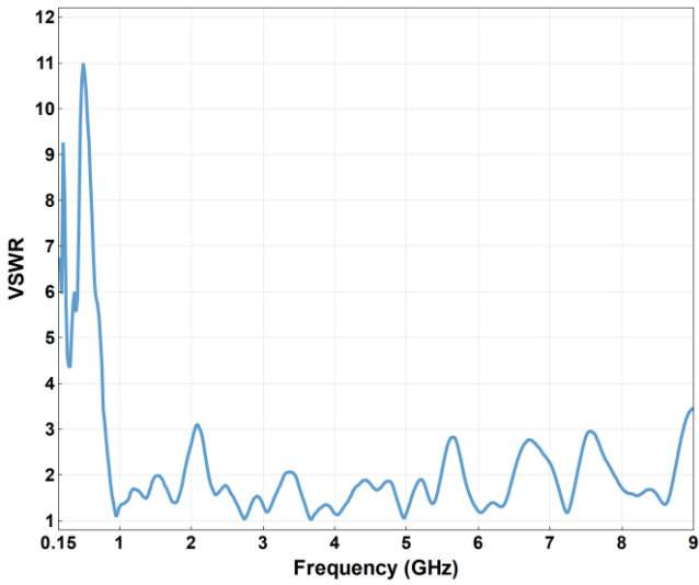
HOA-90 驻波比
