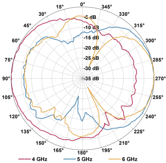
HOA-90 中频段典型方向图
