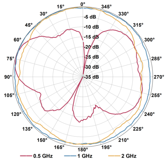
HOA-90 低频段典型方向图
