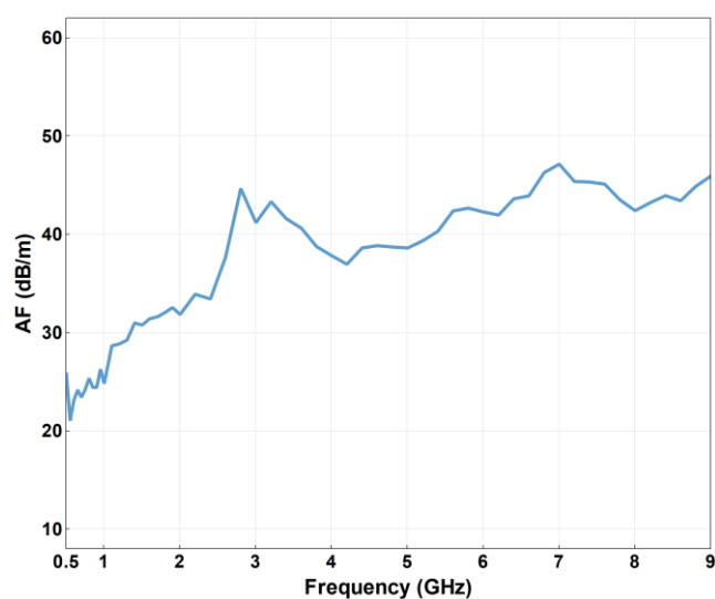
HOA-90 天线因子
