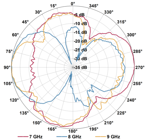
HOA-90 高频段典型方向图
