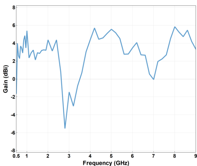
HOA-90 增益
