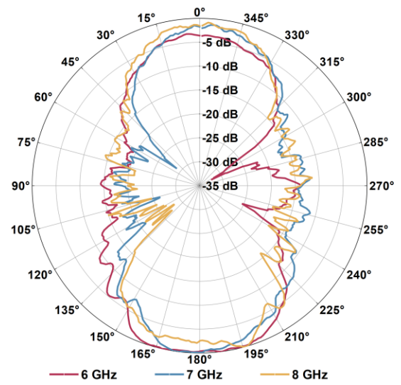
HOA-80 高频段典型方向图
