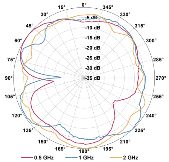
HOA-80 低频段典型方向图
