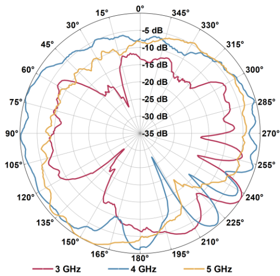
HOA-80 中频段典型方向图
