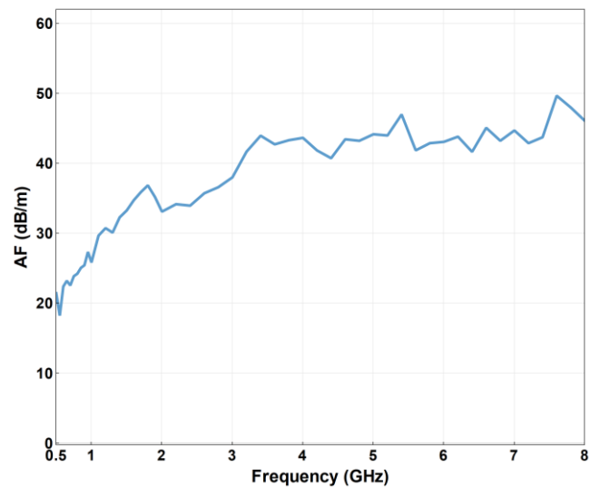
HOA-80 天线因子
