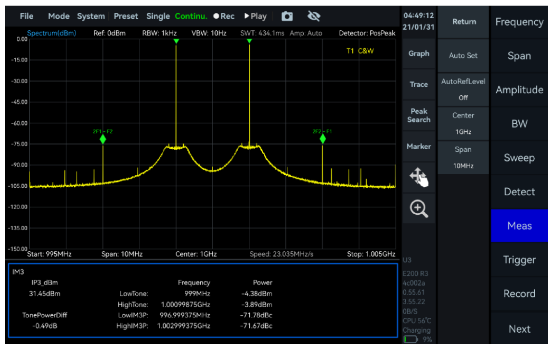
图 21 IP3/IM3 测量
