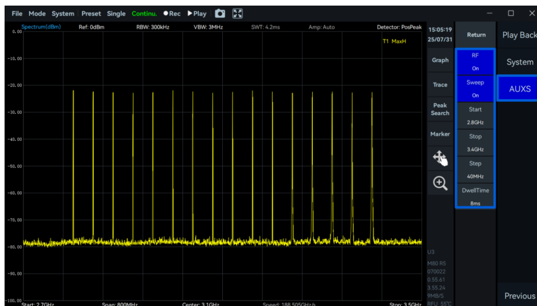
图 40 ASG 输出频率扫描信号
