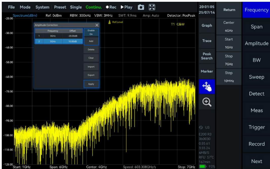
图 17 幅度修正应用
