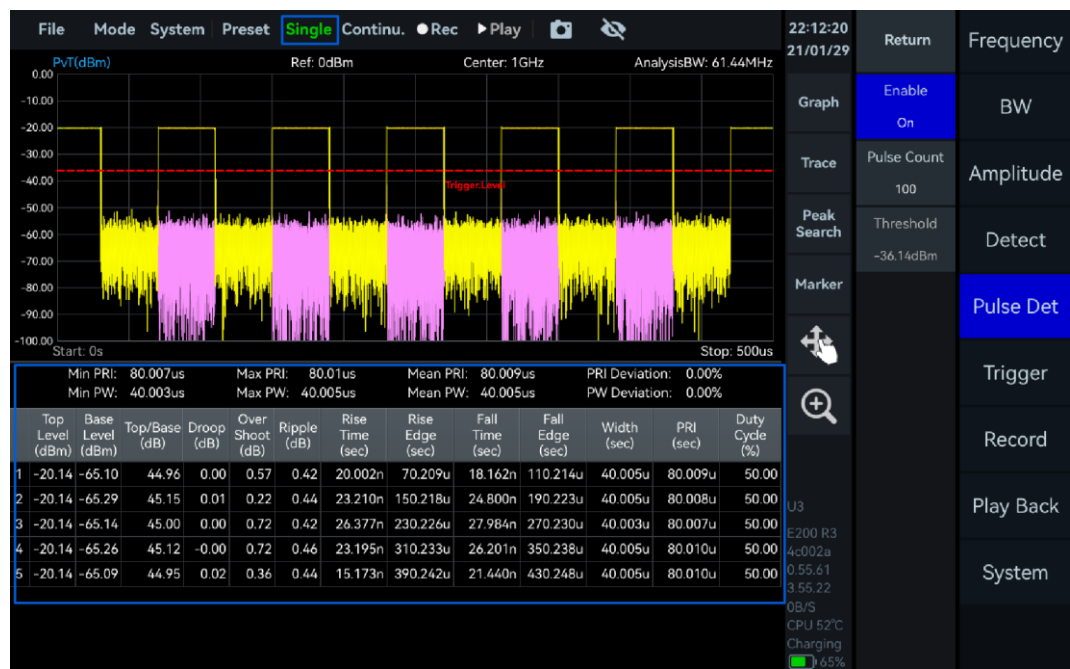
图 32 脉冲检测结果
