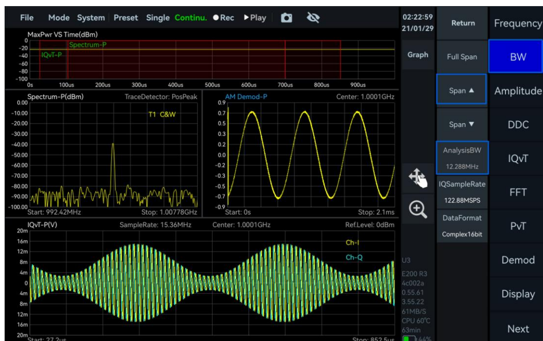
图 26 AM 解调
