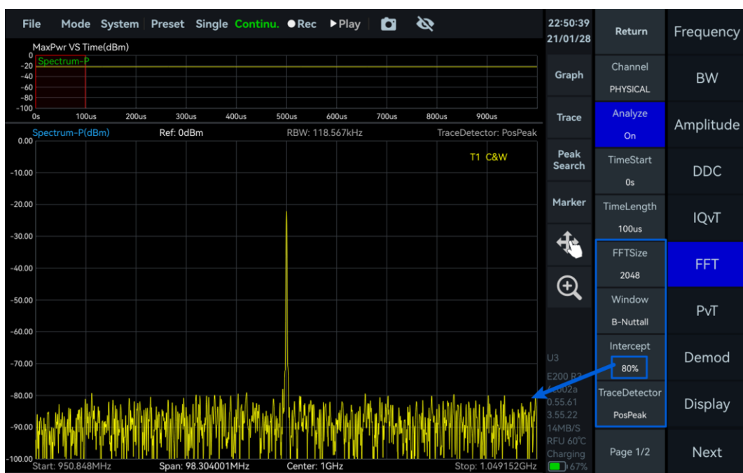
图 23 IQ 数据频谱分析
