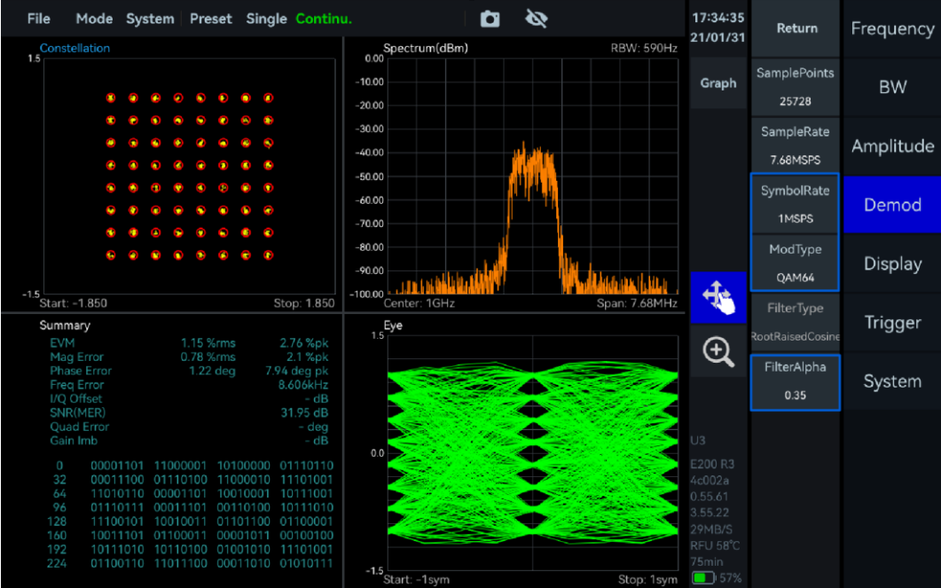
图 35 64QAM 解调
