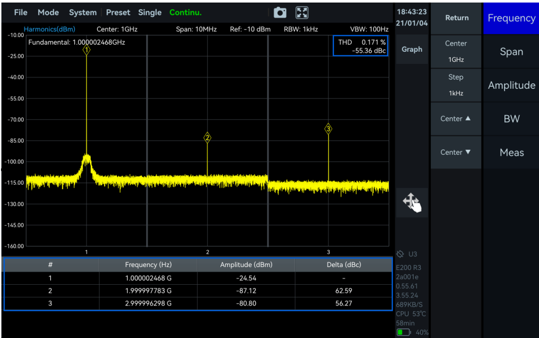
图 36 三次谐波测量
