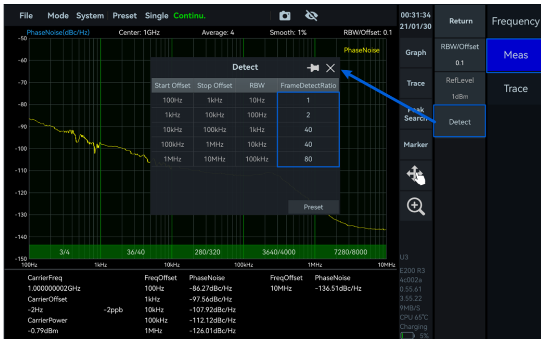
图 37 脉冲信号检测检波设置
