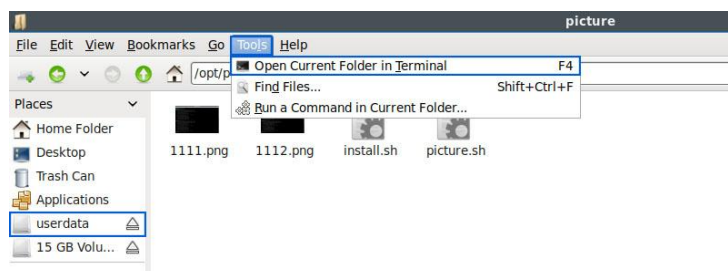
图 44 打开终端
