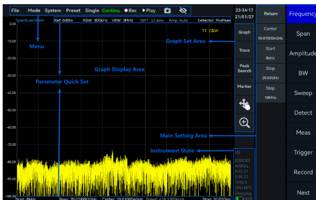
图 3 软件界面布局
