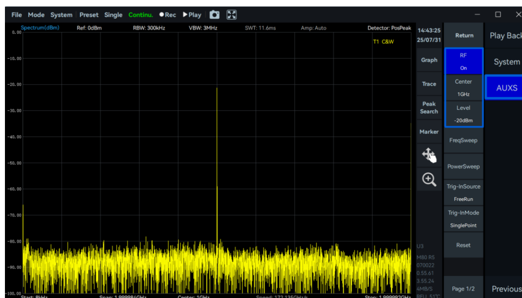
图 39 ASG 输出单音信号
