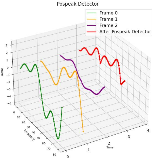
图9 正峰值检波
